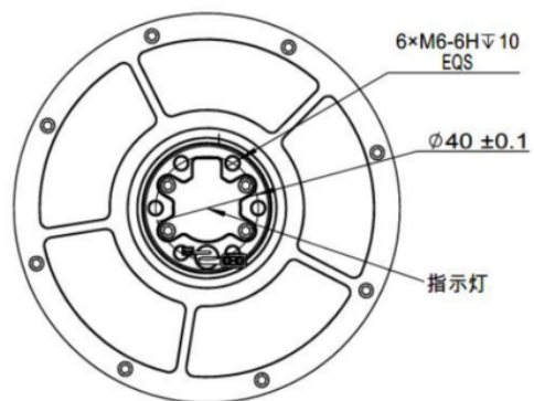
后视图
