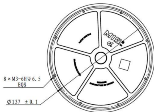
正视图
