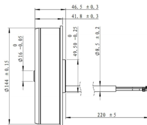
侧视图
