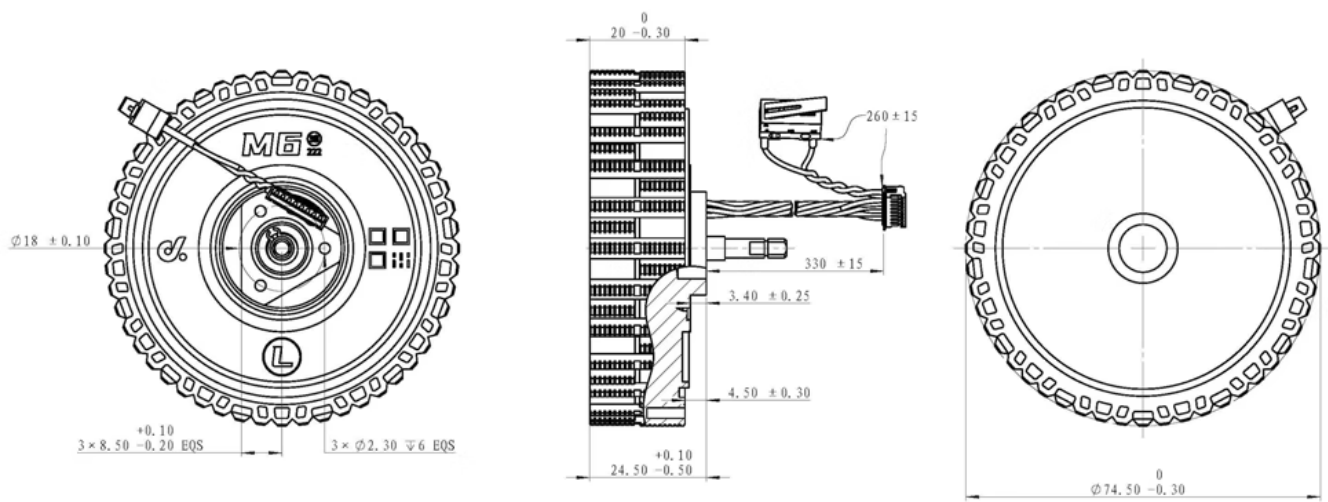
M0603B_224尺寸图
