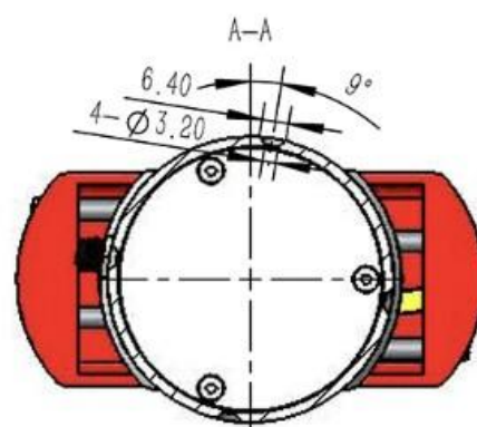
LMG-40夹爪
