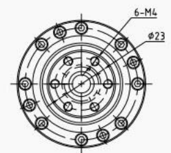
Wave generator-A
