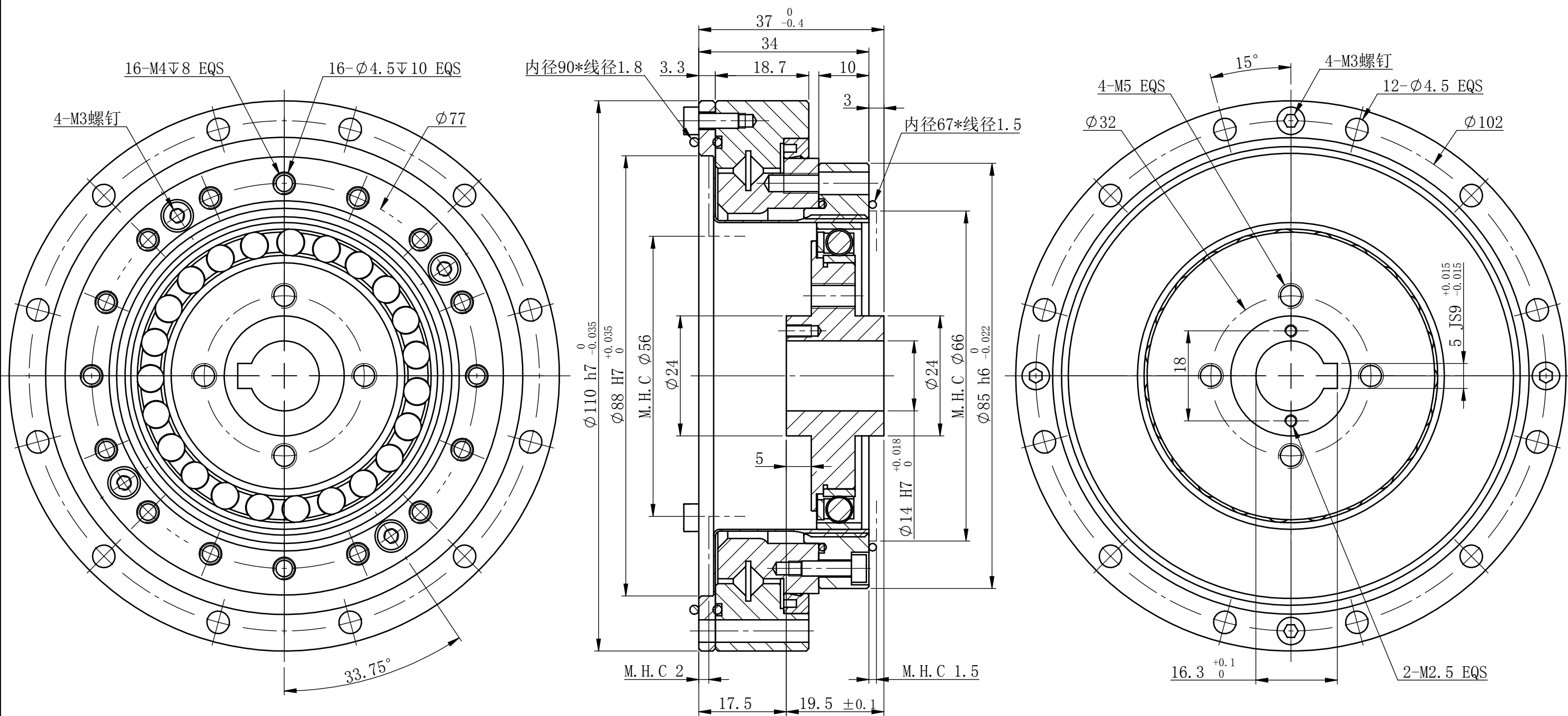
M.H.C:最小安装避让空间 MINIMUM HOUSING CLEARANCE
