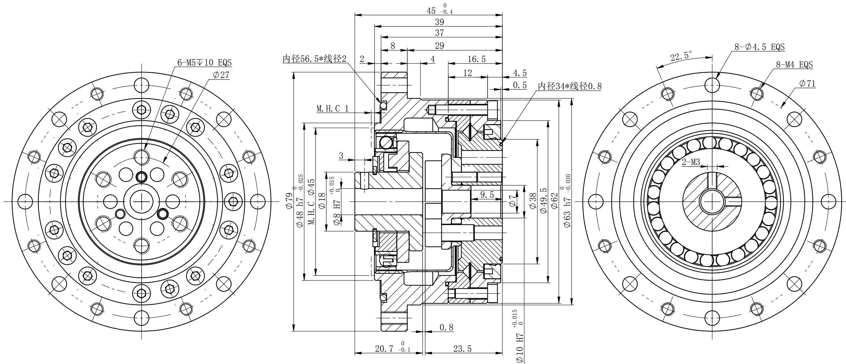
M.H.C :最小安装避让空间 MINIMUM HOUSING CLEARANCE
