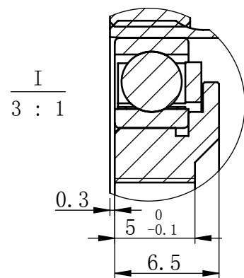
M.H.C :最小安装避让空间 MINIMUM HOUSING CLEARANCE
